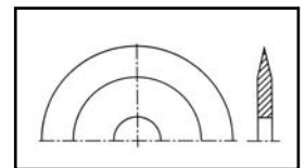
doppelseitige Fase / double side bevel
